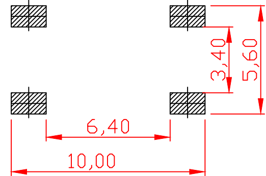
PCB. 焊接图
